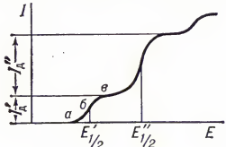
Классическая (постоянноточковая) полярограмма (даны абс. величины значений E ).
